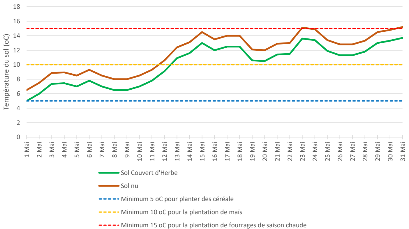
Millstream Température du Sol à 6" de Profondeur
